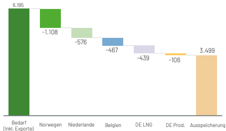
Leistungsbilanz bei 1-tägiger Bedarfsspitze (in GWh/d)
