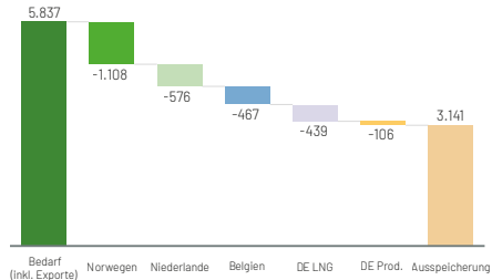
Leistungsbilanz bei 7-tägiger Bedarfsspitze (in GWh/d)
